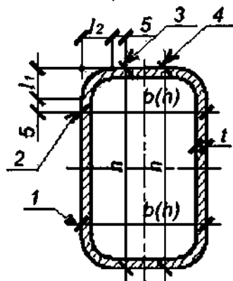
Рисунок 3 – Схема измерения размеров квадратных и прямоугольных профилей
