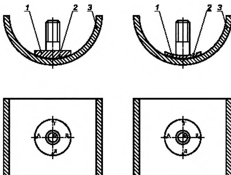
1 — заготовка; 2 — термопластичный клей; 3 — сегмент; А—Д — точки определения толщины слоя клея
